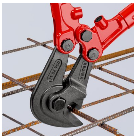
Den speciella huvudformen på armeringsjärnsaxen 71 82 950 gör det möjligt att klippa planliggande byggnadsstål
